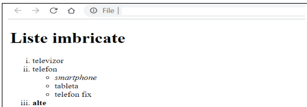
Fig.1.12. Rezultatul obținut la vizualizarea paginii WEB într-un browser.
